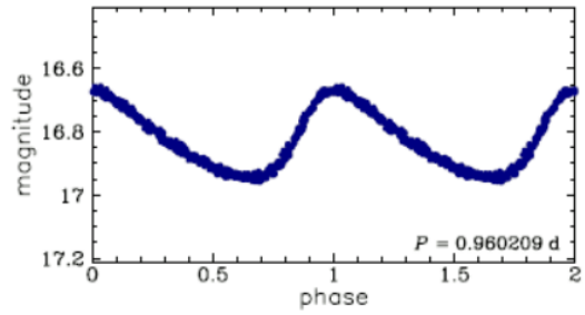
Figura 11: Curva de magnitud con respecto a fase de una ceféida clásica oscilando en el primer armónico. Vemos que no hay progresión de Hertzsprung y que la amplitud de la oscilación es menor que para una estrella en el modo fundamental.
